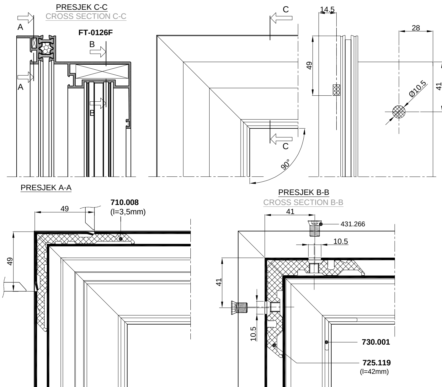
PRESJEK A-A CROSS SECTION A-A
