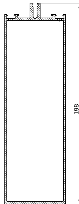
PRESJEK B-B CROSS SECTION B-B
