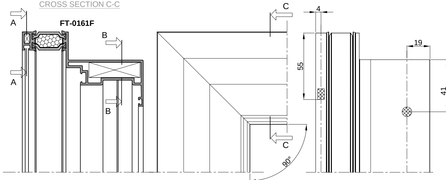
PRESJEK C-C CROSS SECTION C-C
