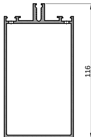
PRESJEK B-B CROSS SECTION B-B
