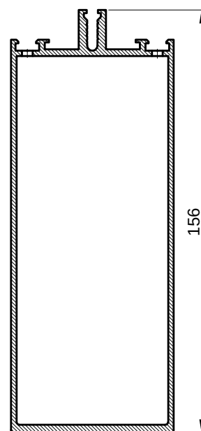
PRESJEK B-B CROSS SECTION B-B
