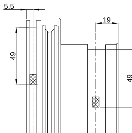
PRESJEK B-B CROSS SECTION B-B
