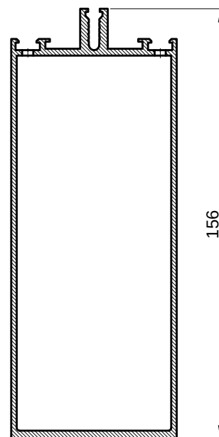
PRESJEK B-B CROSS SECTION B-B
