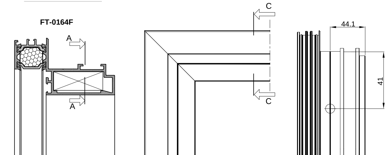
PRESJEK C-C CROSS SECTION C-C
