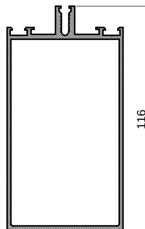
PRESJEK B-B CROSS SECTION B-B
