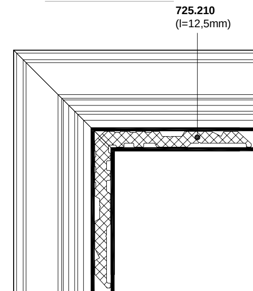
PRESJEK B-B CROSS SECTION B-B
