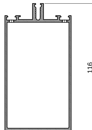
PRESJEK B-B CROSS SECTION B-B
