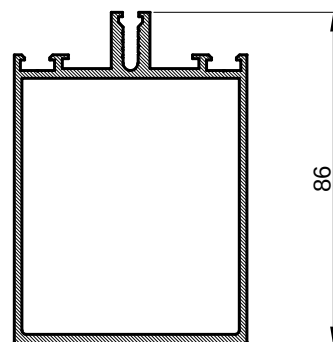
PRESJEK B-B CROSS SECTION B-B
