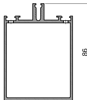
PRESJEK B-B CROSS SECTION B-B
