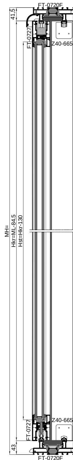
KLIZNA I PODIZNO-KLIZNA DVOKRILNA VRATA SA KRILOM FT-0727 SLIDE AND LIFT-SLIDE TWO SASH DOOR WITH SASH FT-0727
