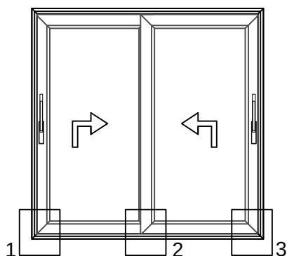
Ugradnja profila: FT-0734F
