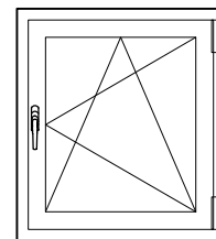
Skriveno krilo Hidden sash
