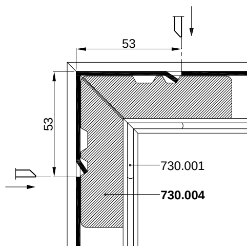
PRESJEK C-C
