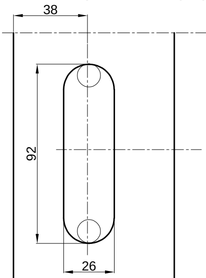
POGLED Obrada za vanjski rukohvatnik VIEW Processing for external finger grip
