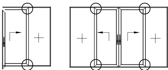
UGRADNJA UBLAŽIVAČA UDARA KRILA 345.010
