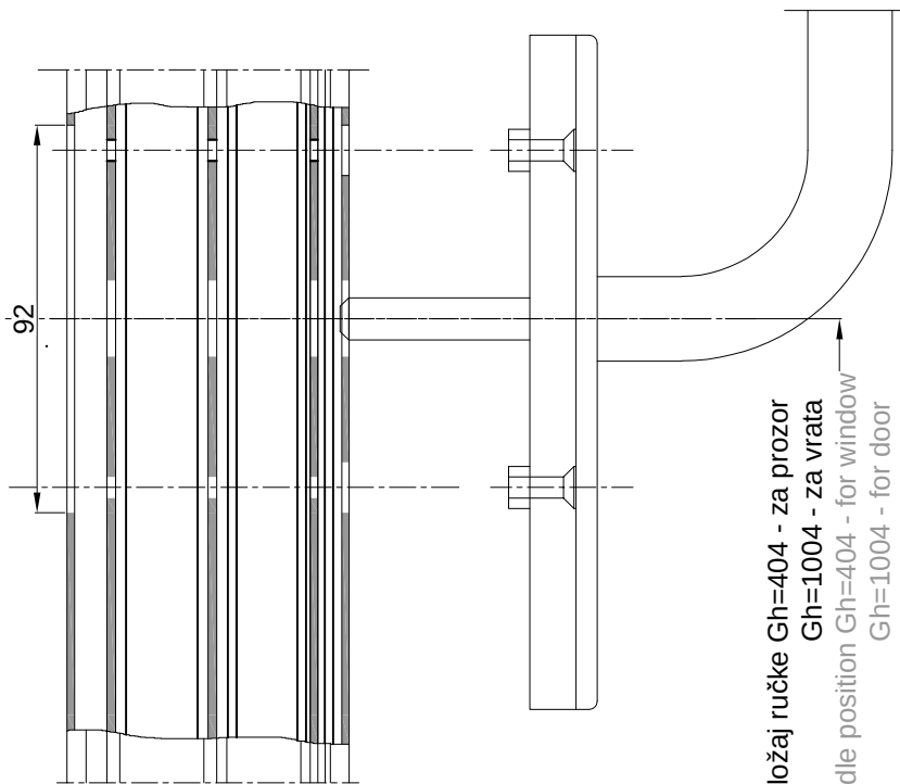
PRESJEK D-D CROSS SECTION D-D
